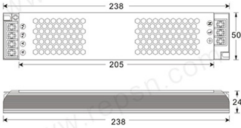
RPS-400HL-12
