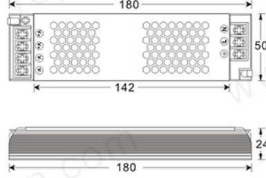
RPS-200HL-12
