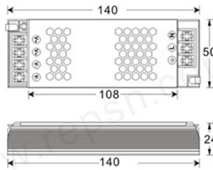
RPS-100HL-12
