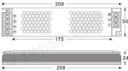
RPS-300HL-12
